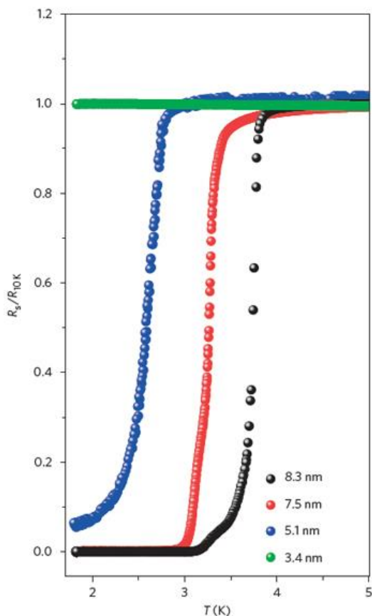
Рис. 2. Температурные зависимости электросопротивления пленок \text{Mo}_2\text{C} различной толщины.
