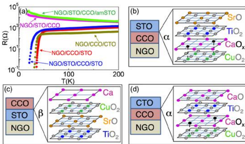
а – Температурные зависимости сопротивления двухслойных и трехслойных пленок из слоев \text{CaCuO}_2 (CCO), \text{SrTiO}_3 (STO) и \text{CaTiO}_3 (CTO) на подложках \text{NdGaO}_3 (NGO). Здесь amSTO – аморфный слой \text{SrTiO}_3 . б-д – Схематическое изображение структуры различных границ раздела.
