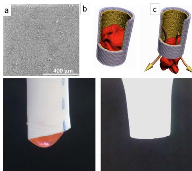
Рис. 3. (a) SEM изображение тромболитического золь-гель покрытия на стенке сосудистого графта. Схема (b,c) и фотографии процесса растворения и удаления искусственного тромба из графта с покрытием. В графте без покрытия (внизу) тромб полностью сохранился.
