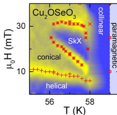
Рис. 1. Фазовая диаграмма \text{Cu}_2\text{OSeO}_3 : SkX – решетка скирмионов [2].
